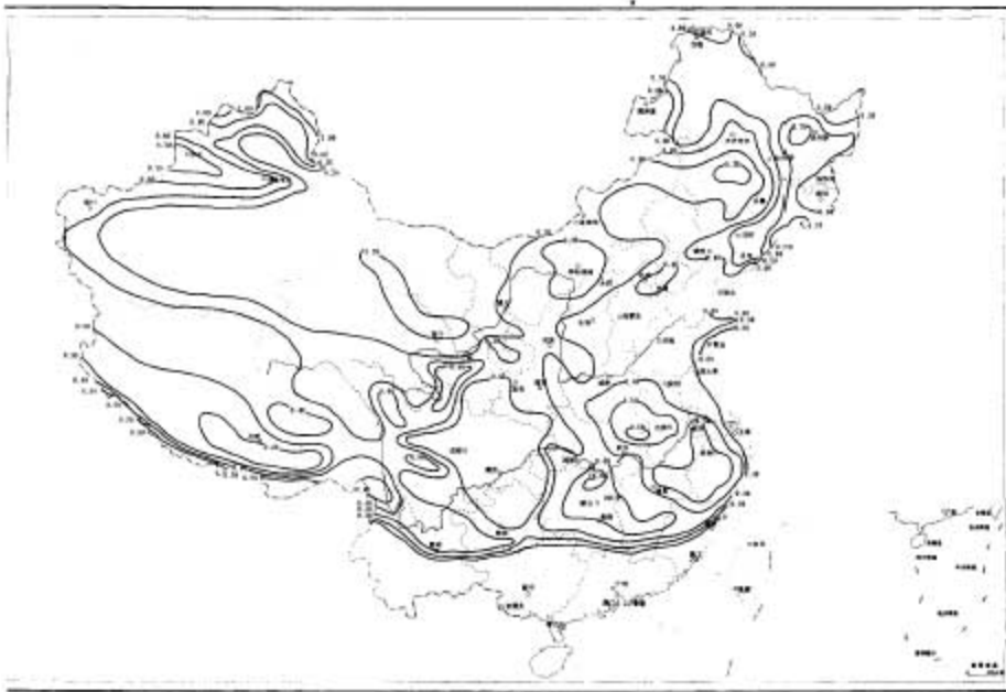
图 2.1.1 中国最暖月(7月)等温线图
