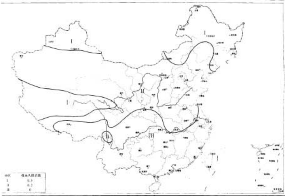
图 2.1.2 中国各月无霜期日数分布图
